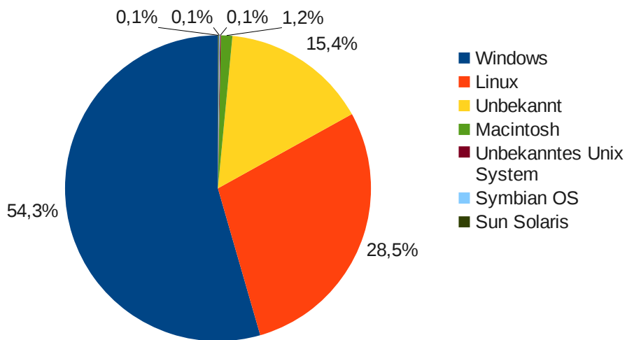
benutzte Betriebssysteme
