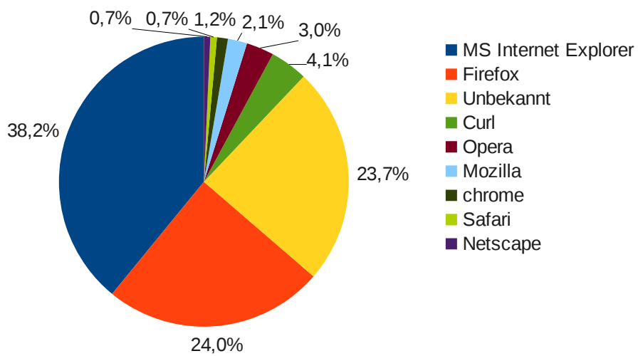
benutzte Browser
